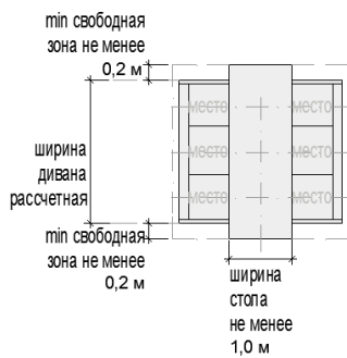
взаиморасположение мебели и проходы:
