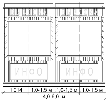
главный фасад и задний фасад (просем открыт)
