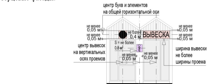
главный фасад: торцевые фасады:
